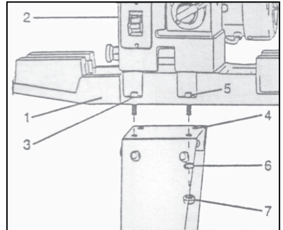
Фигура 15 – стабилизиране на основата
