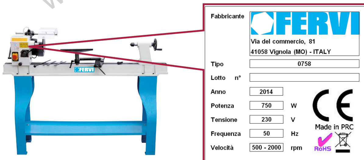
Фигура 8 – Идентификационна табелка за 0758
