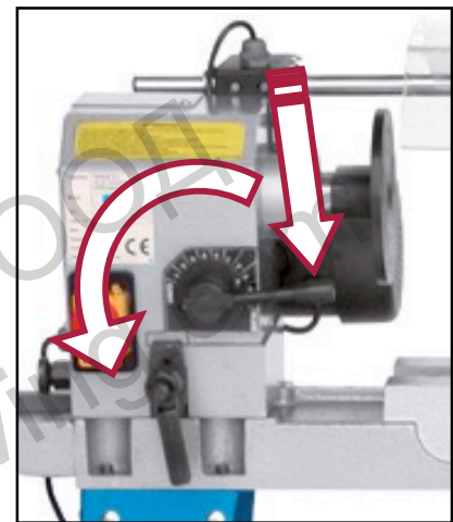
Фигура 17 – избиране на скорост.
