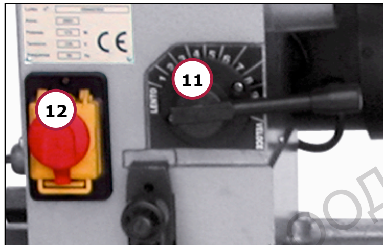
Фигура 7 – пулт за управление
