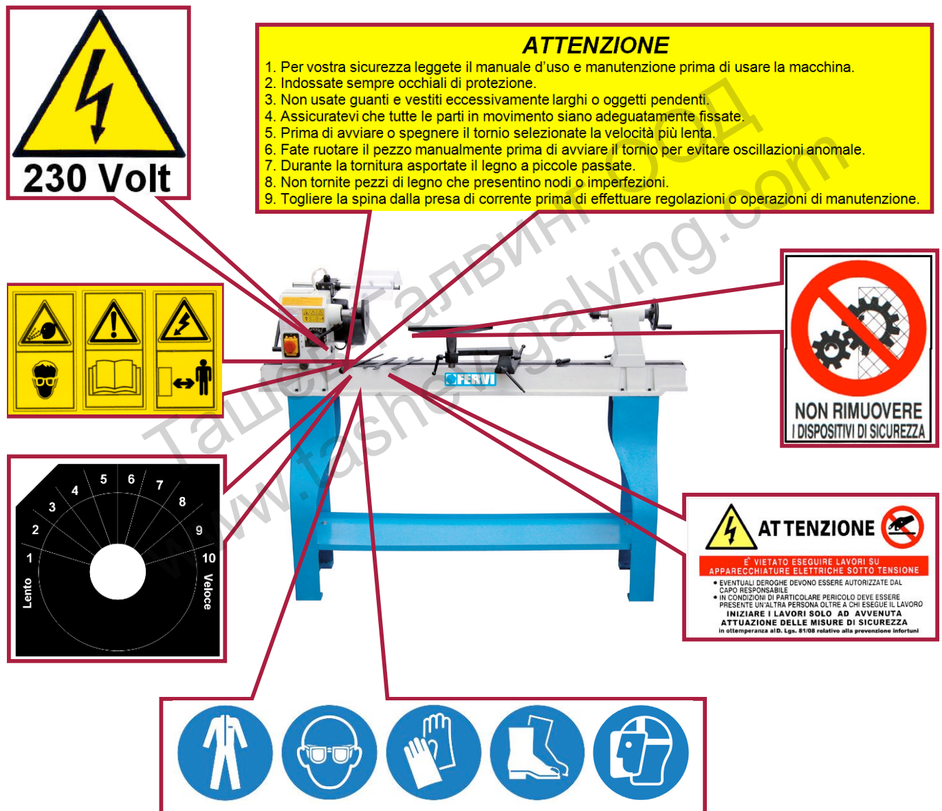
Фигура 9 – табелки и пиктограми, прикрепени към машината.
