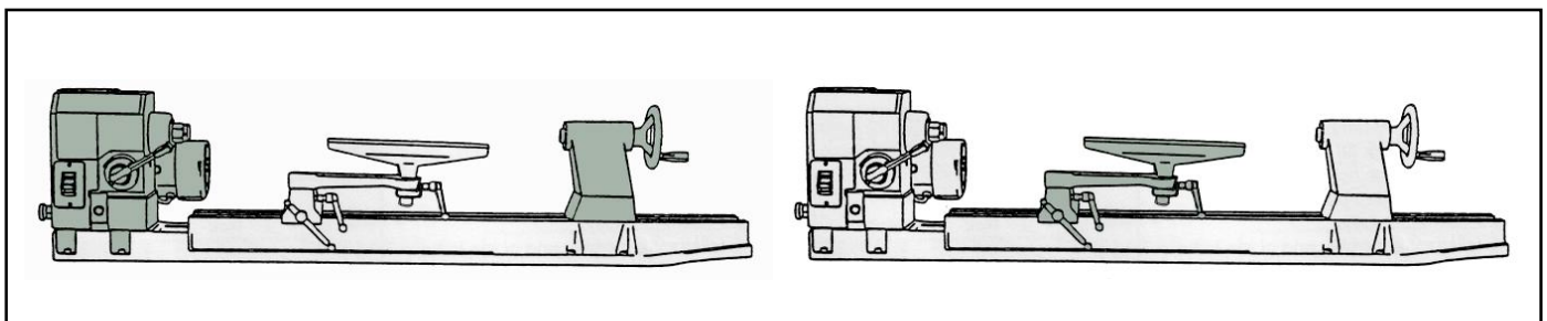
Фигура 1 – основни части на струга за дърво
