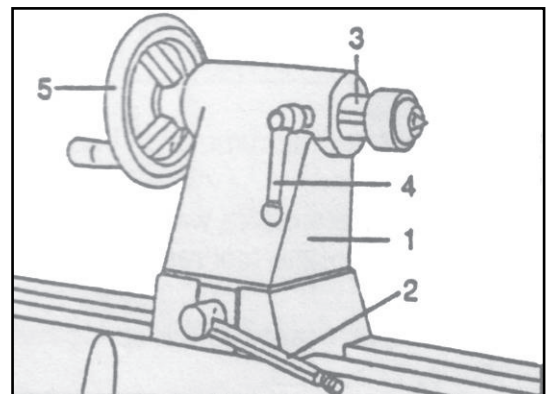
Фигура 19 – задно седло
