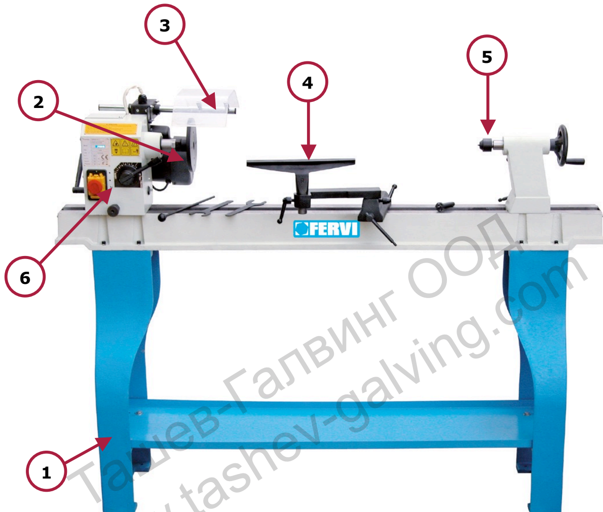
Фигура 2 – основни части на струг за дърво 0758
