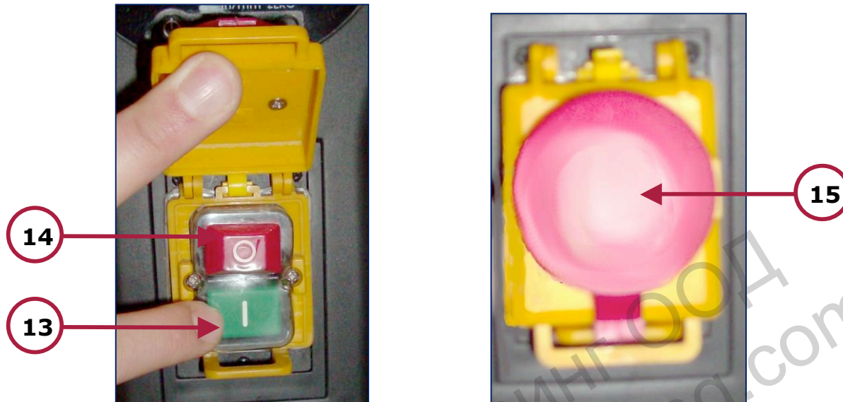
Фигура 16 – бутон за стартиране/спиране и аварийно спиране
