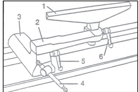
Фигура 18 – държач на инструмента
