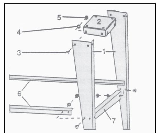
Фигура 14 – местоположение на точките на свързване
