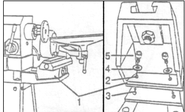
Фигура 23 – конфигурация с удължител
